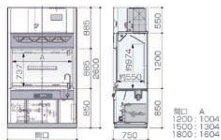
尺寸图 (mm)
