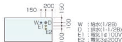
尺寸图 (mm)
