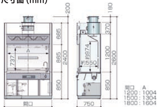
尺寸图 (mm)
